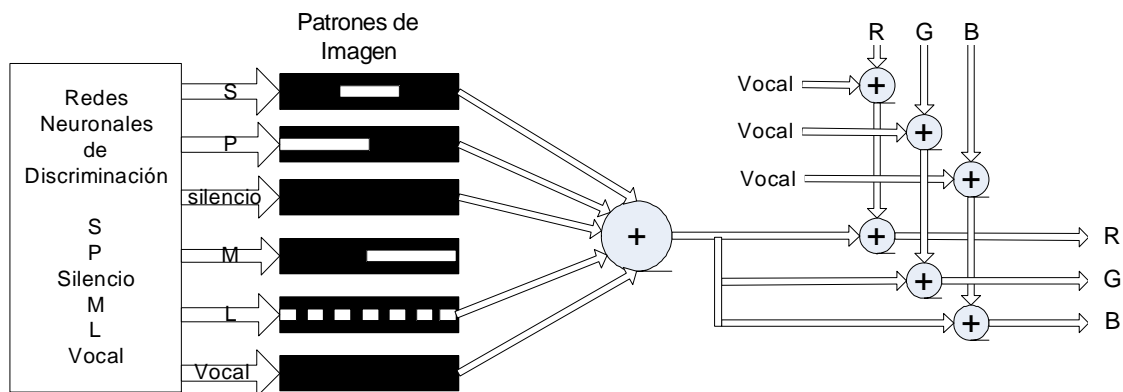
Figura 3 Esquema de la unidad sintetizadora de imagen
