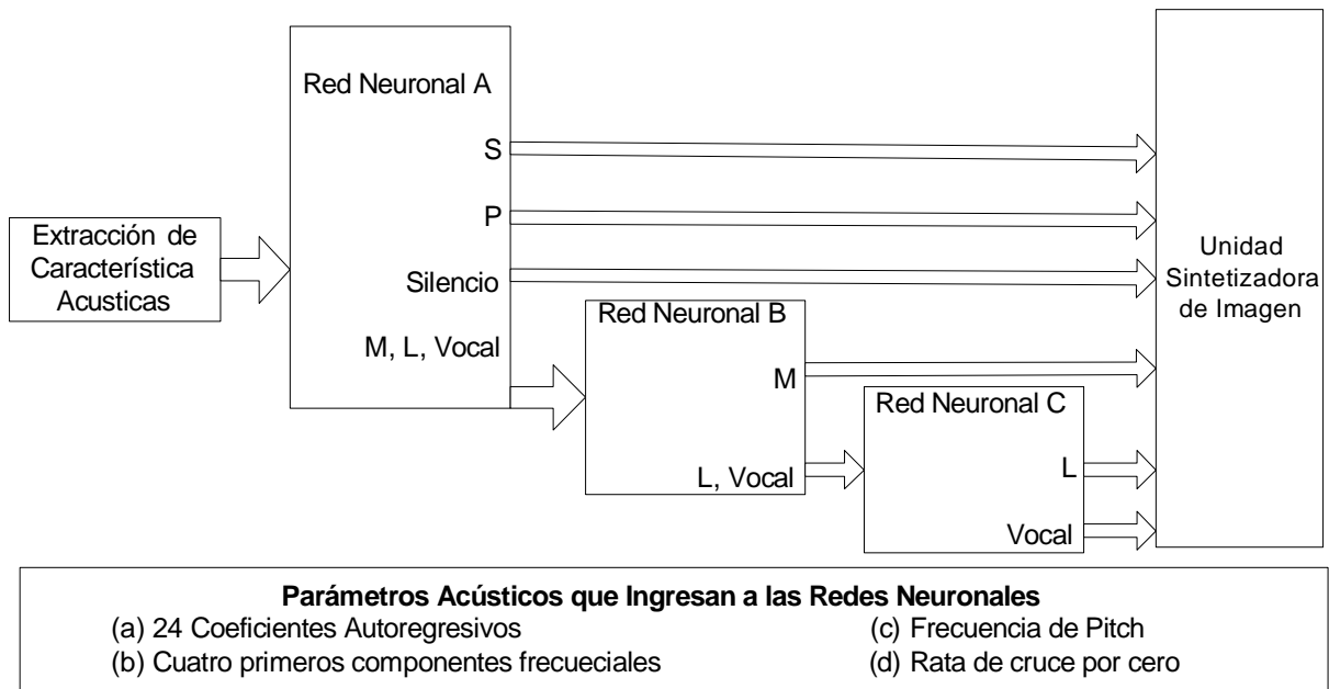
Figura 2 Redes Neuronales de discriminación
